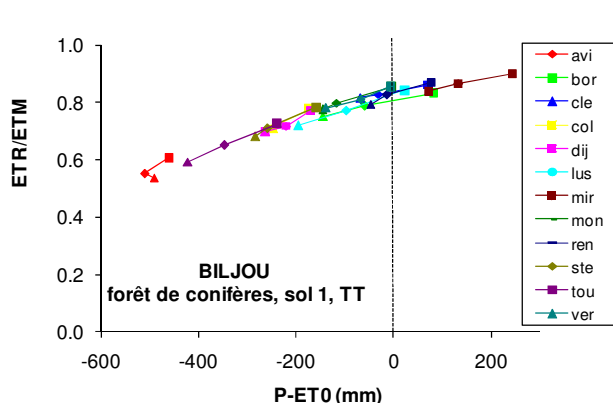
Figure 1 : Evolution avec BILJOU du rapport ETR/ETM pour les conifères en fonction de l'indice agroclimatique ( P-ET0 : ■ passé récent, ♦ futur proche, ▲ futur lointain)
