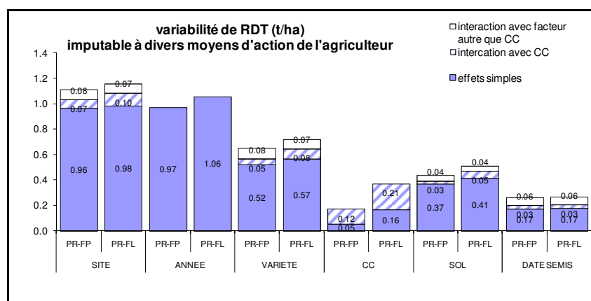
Figure 2 : analyse de la variance pour le rendement de blé simulé avec PANORAMIX. Pour chaque facteur, en bleu uni la part de variance correspondant à l'effet simple ; en bleu hachuré, la part de l'interaction avec la période (CC) ; en transparent, la part de l'interaction avec d'autres facteurs que la période. Le CC a été considéré séparément pour l'horizon proche (FP) et l'horizon lointain (FL).
