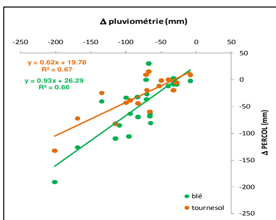
Figure 5 : Baisse de la recharge des aquifères en fonction de la baisse de pluviométrie pour le tournesol (orange) et le blé (vert).
